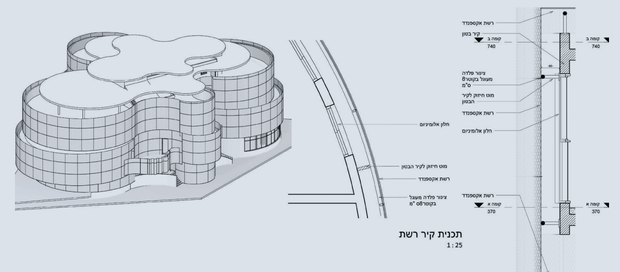
אפשרות עיגון לבטון ללא קורה מעורגלת
